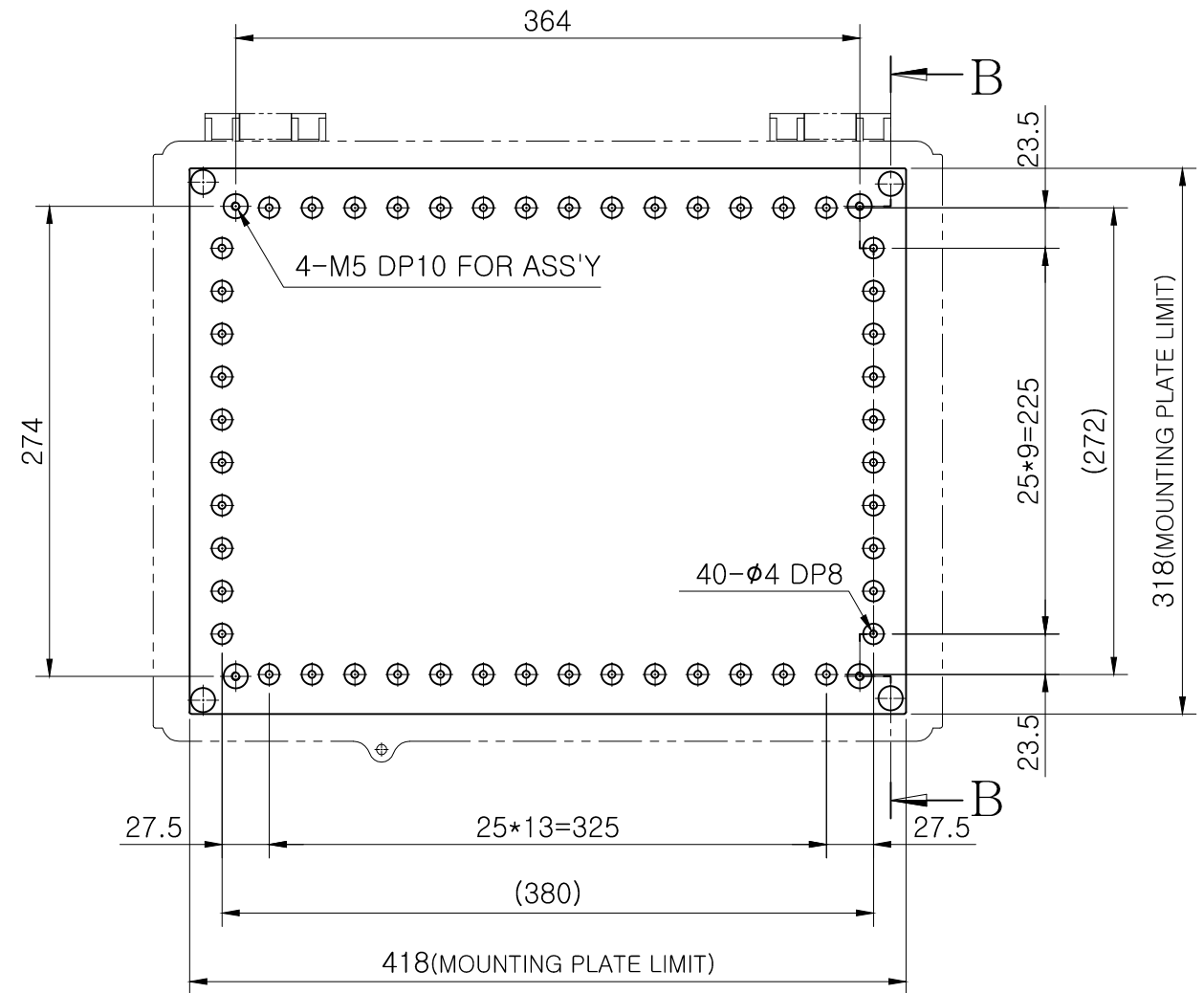
SECTION A-A
