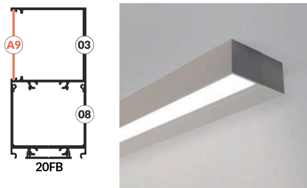
variant 32 - wall side 20FB-08-03-A9 wariant 32 - ścienny boczny 20FB-08-03-A9
