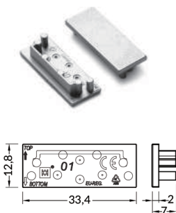
VARIO 01 End Cap
