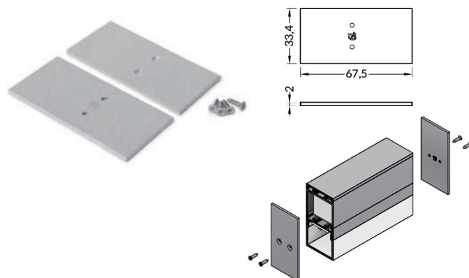
VARIO 19 Metal End Cap
