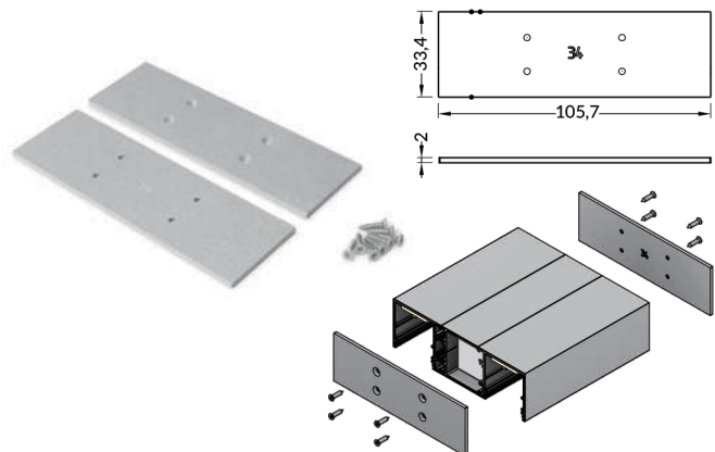
VARIO 34 Metal End Cap
