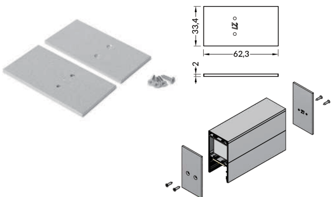
VARIO 27 Metal End Cap
