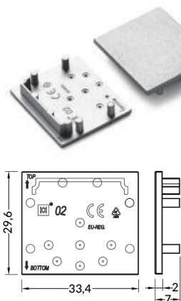
VARIO 02 End Cap
