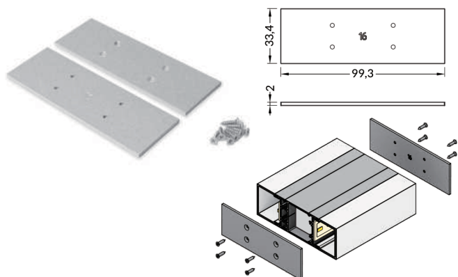
VARIO 16 Metal End Cap
