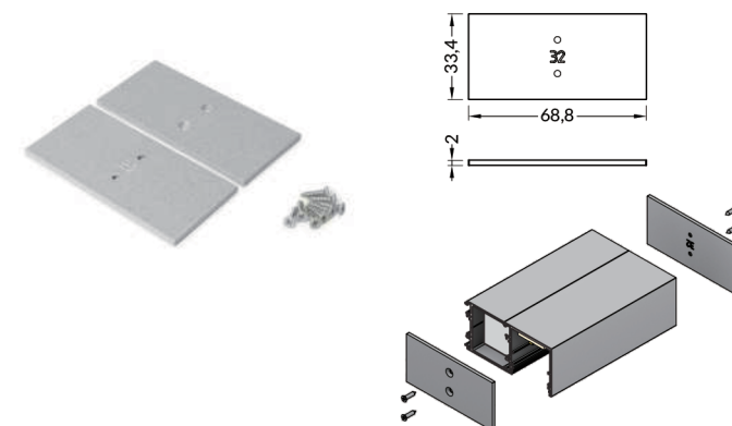
VARIO 32 Metal End Cap
