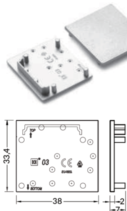
VARIO 03 End Cap
