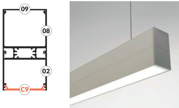
variant 27 - pendant 09-08-02-C9 wariant 27 - wiszący 09-08-02-C9
