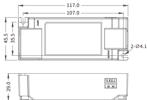
DUL060-B
