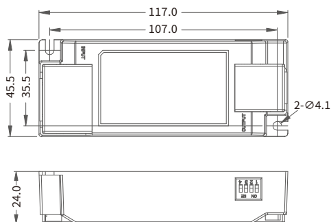
DUL010-B
