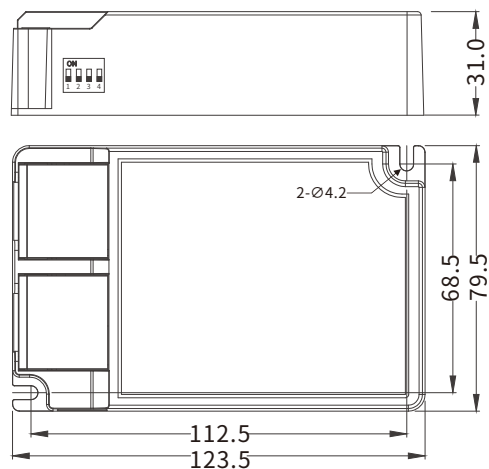
DUL060-B
